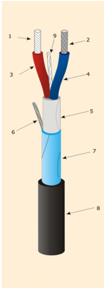
ATHC 双芯发热电缆结构图
